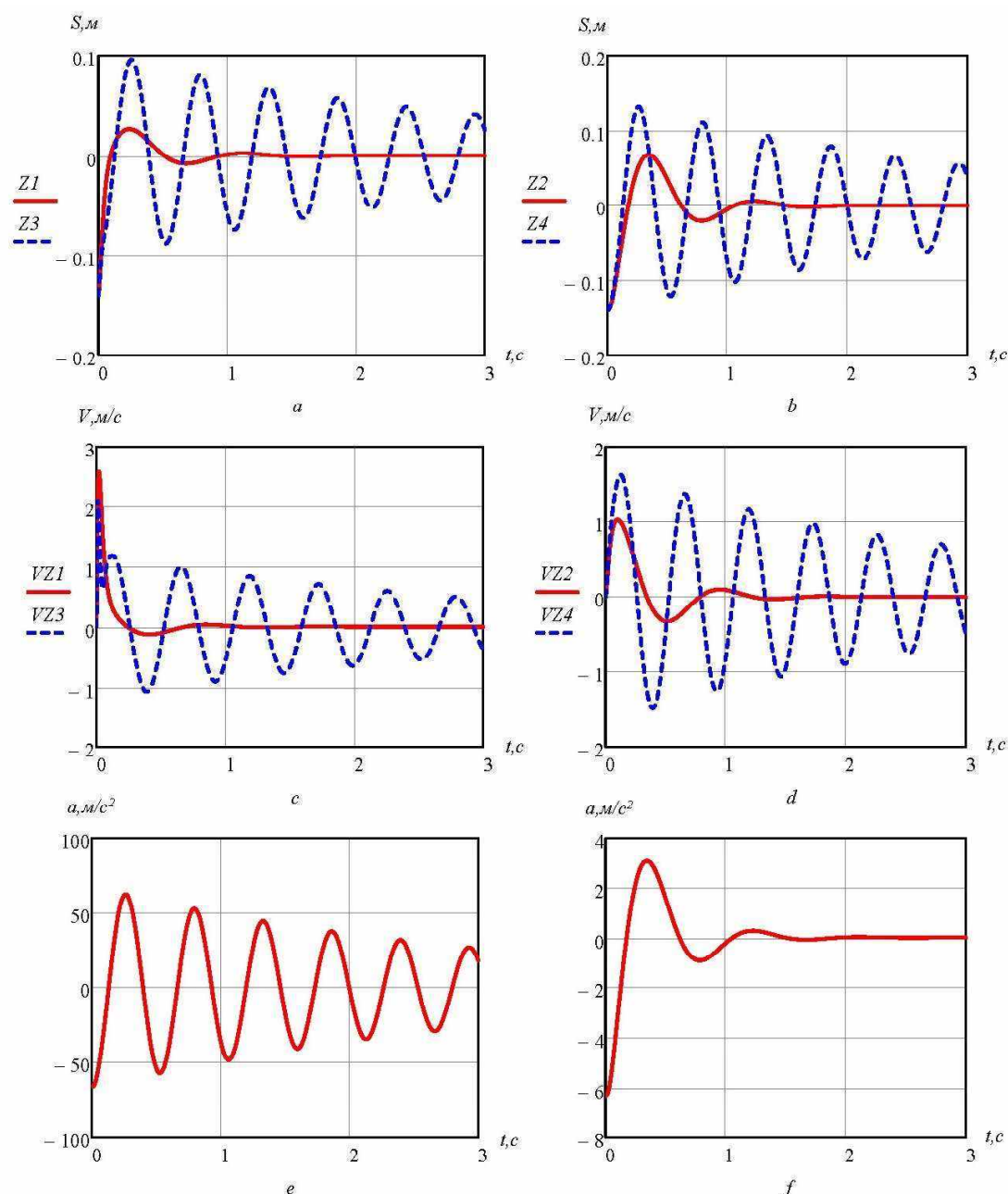
Рис. 4. Результаты моделирования в MathCAD изменения характеристик колебательного процесса поддрессоренной и недрессоренной массы автомобиля по времени t (сек), полученные проезда неровности высотой 0,14 м:
