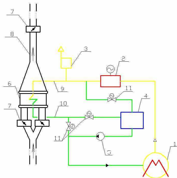
Рис. 1. Принципиальная схема модернизированной СПОТ ПГ:
