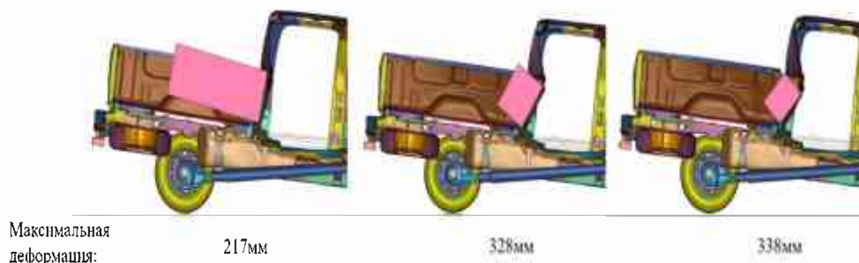
Рис. 7. Перемещения стенки при ударе блоков разных габаритов
