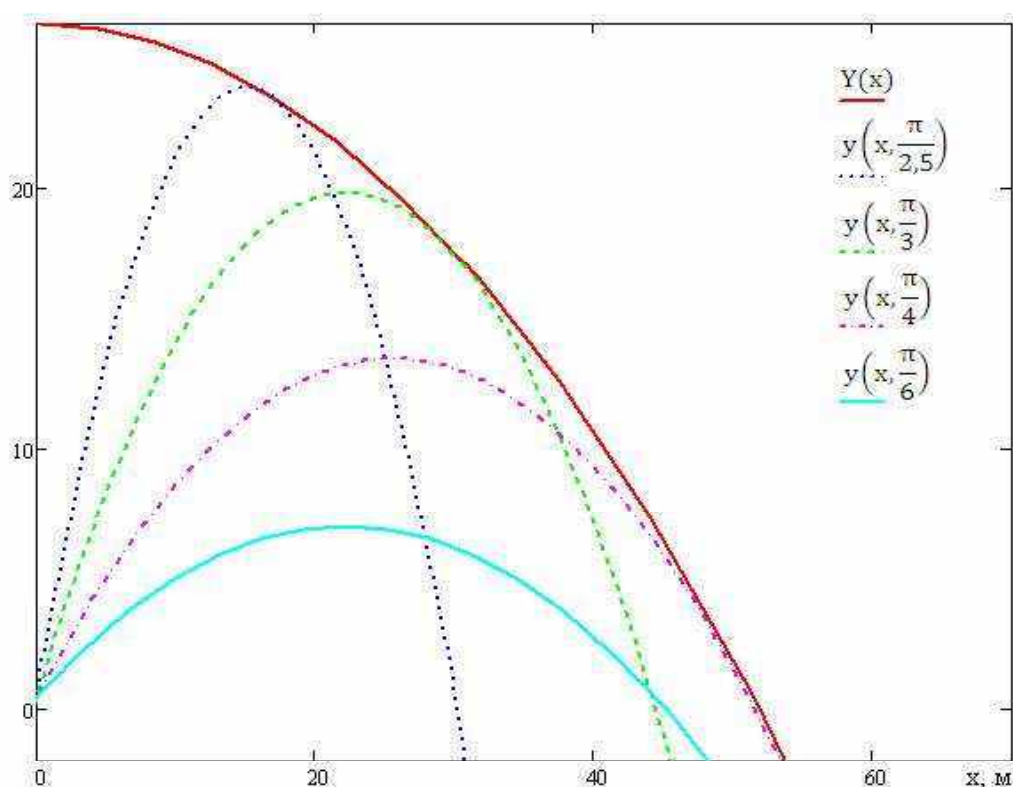
Рис. 4. Огибающая и частные траектории полета крышки арматуры
